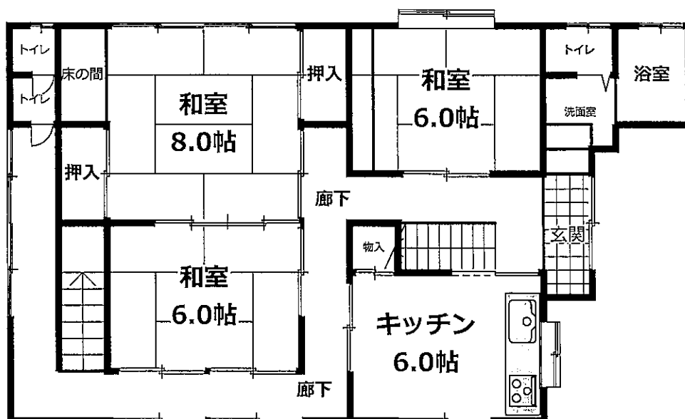
1 階 縮尺 1/100
