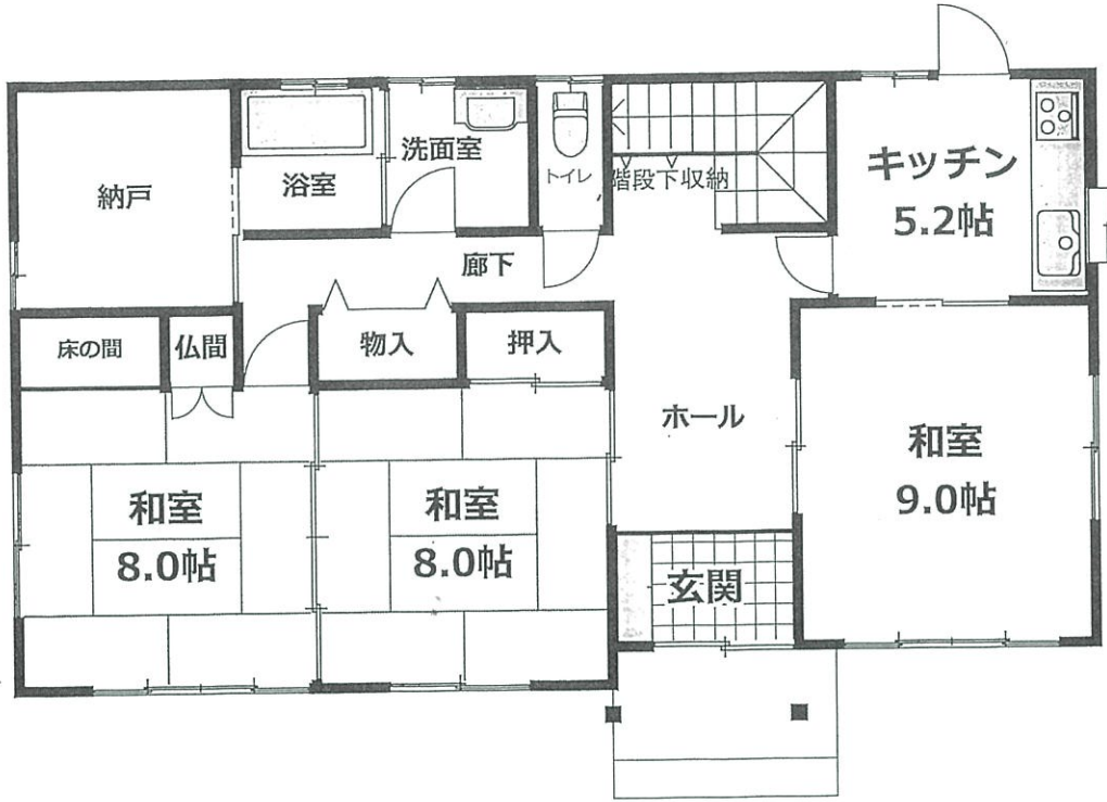
1階 縮尺 1/100
