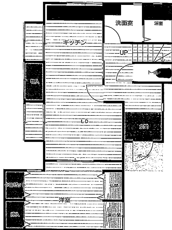
1階縮尺 1/100
